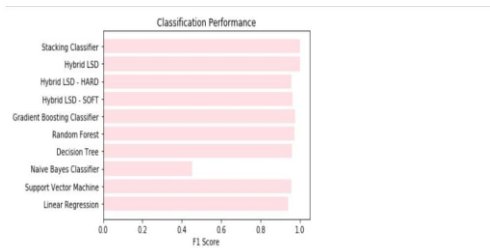
Fig 16 F1Score
