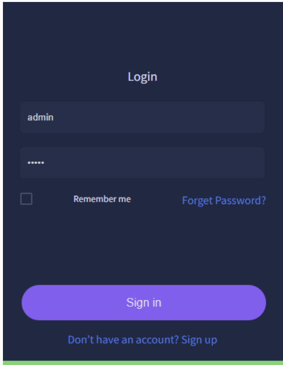
Fig 20 Login page
